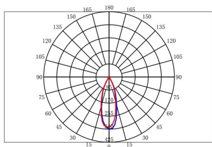
配光曲线
